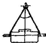
Схема строповки вкладыша
