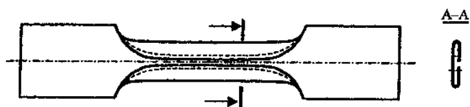
Рис. 7б. Сложенная петля — исполнение «Б»
