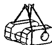
Схема строповки детали пресса
